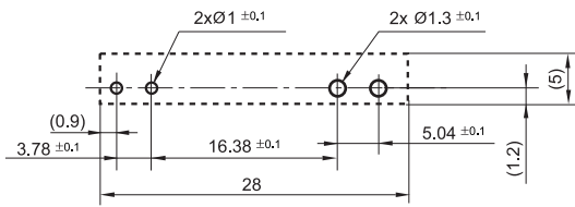
垂直安装型
