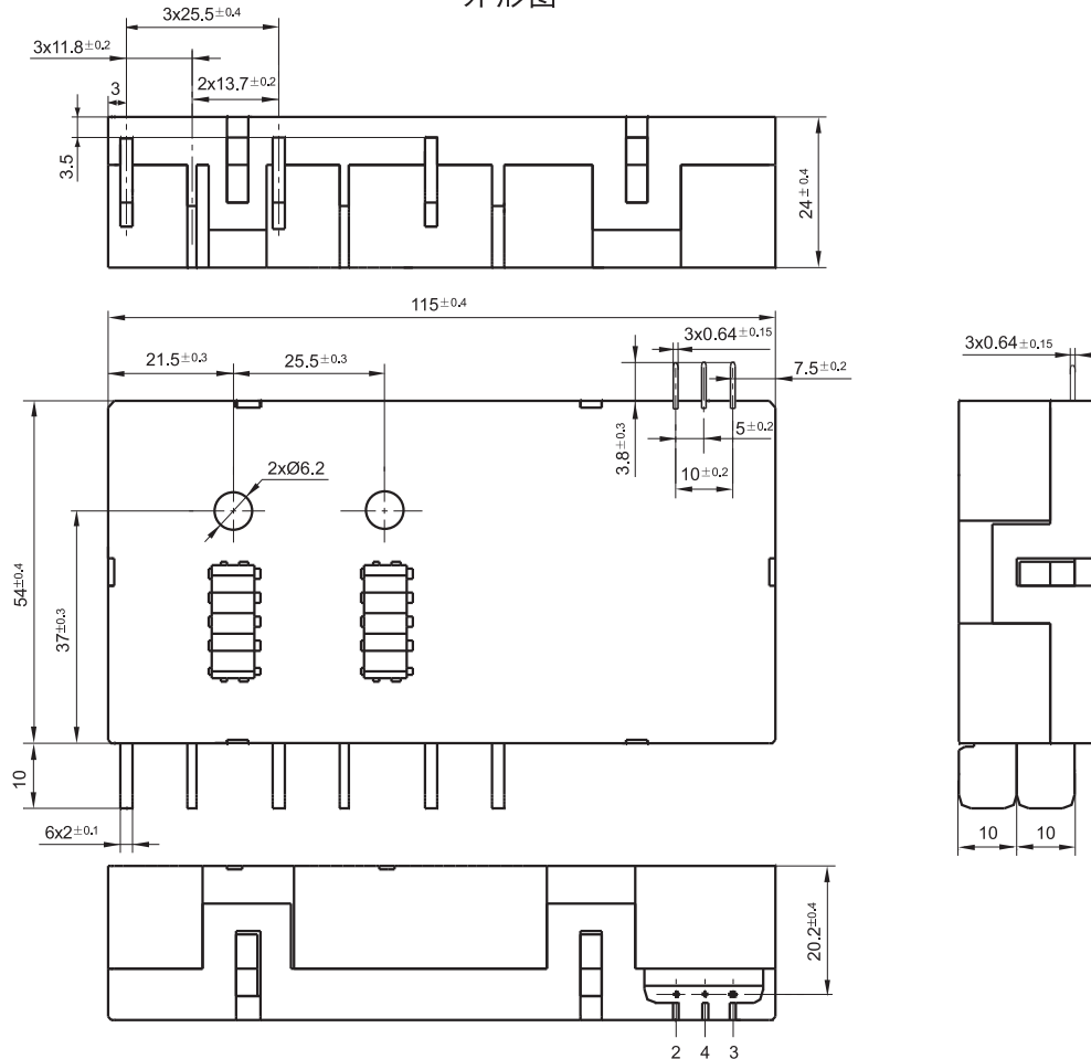
外形图
